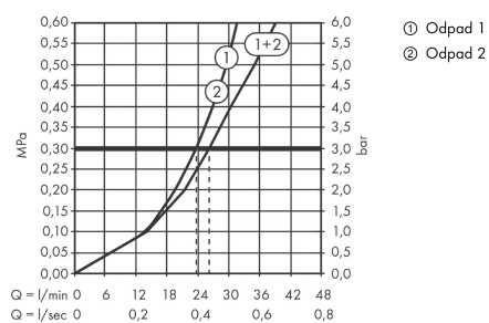
Průtokový diagram
