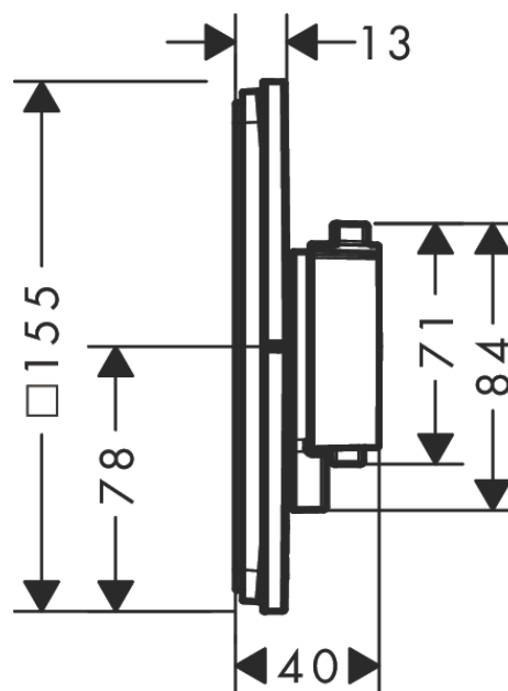
Kótovaný výkres
